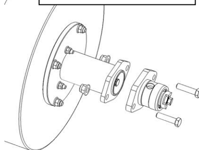
Kupplungsanschluss
